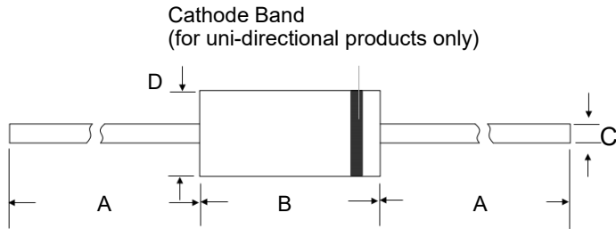
DO - 201
